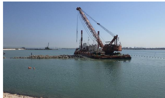
▲ 捨石の投入（仮締切堤）
