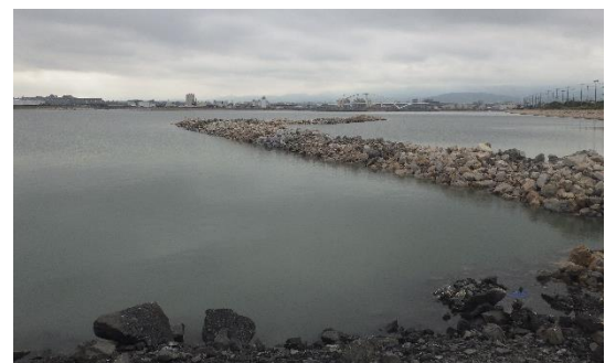
▲ 仮締切堤全景
