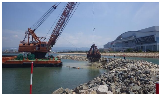
▲ 捨石の投入
